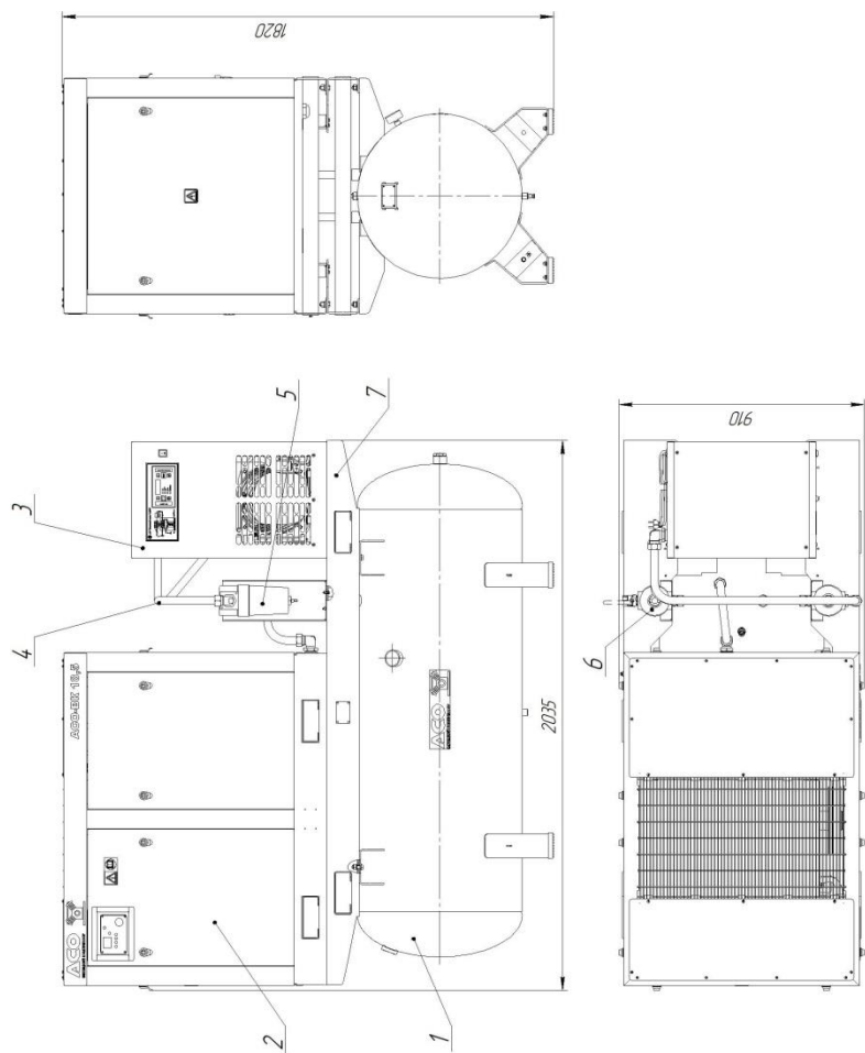
Рисунок 1. Установка компрессорная ВК-18.5М2-ОБ-500 1 – ресивер, 2 – агрегат компрессорный, 3 – осушитель воздуха 4 – система трубопроводов, 5 – фильтр магистральный АС1041 6 – фильтр магистральный АС1043, 7 – плита установочная
